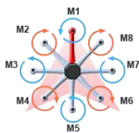
Octo-rotor I
